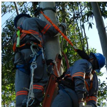
Figura 47 – Socorrista passando o talabarte de posicionamento
