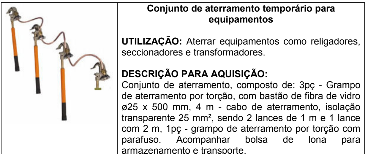
Figura 64 – Conjunto de aterramento temporário para equipamentos
