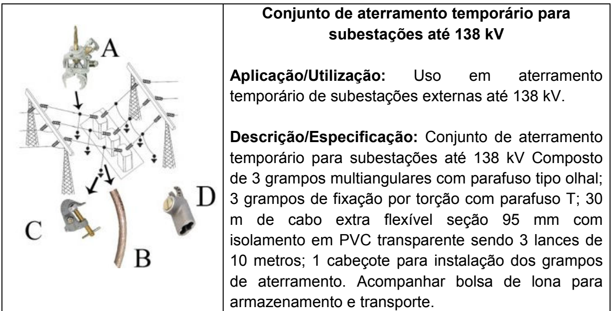
Figura 63 – Conjunto de aterramento temporário para subestações até 138 kV
