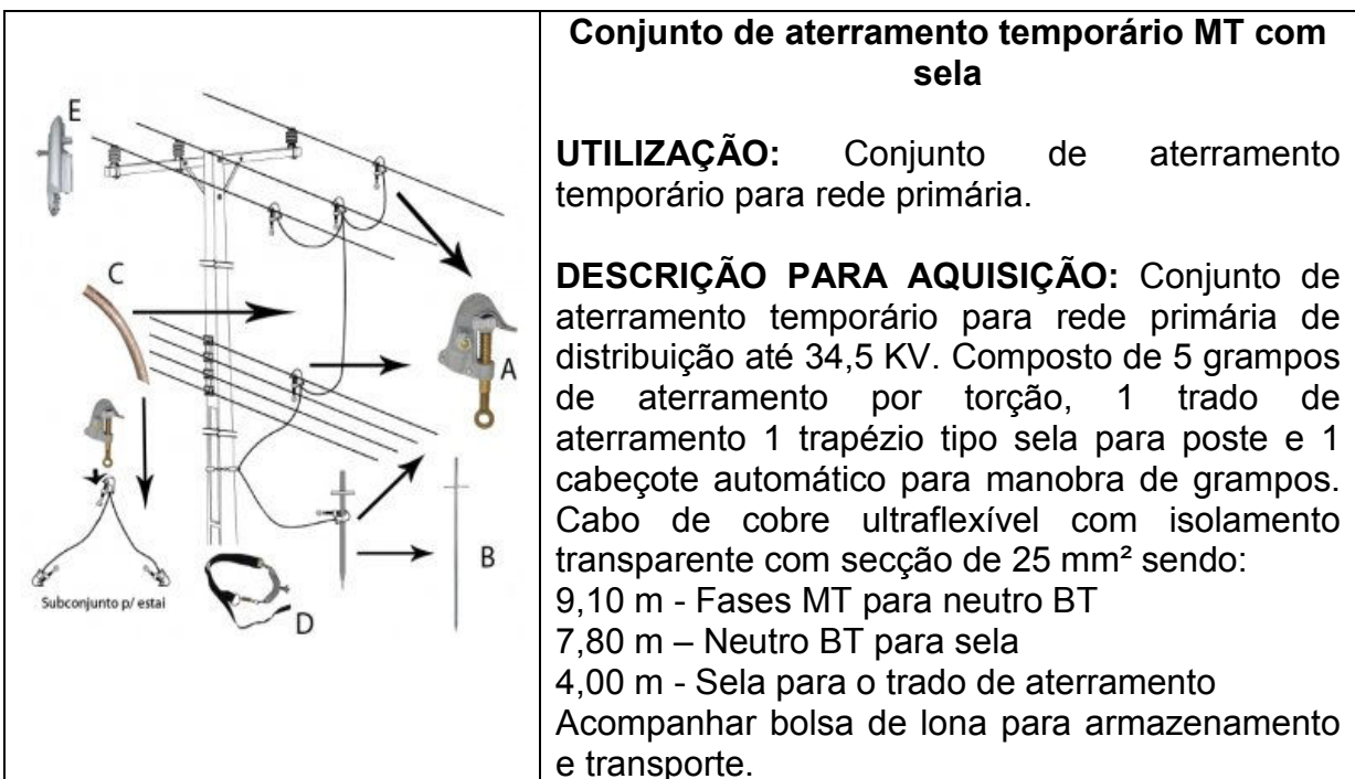
Figura 62 – Conjunto de aterramento temporário MT com sela
