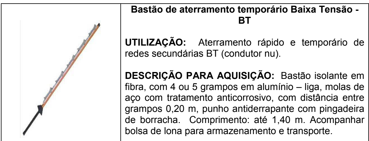
Figura 65 – Bastão de aterramento temporário BT.
