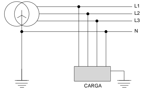
Figura 4 - Esquema TT
